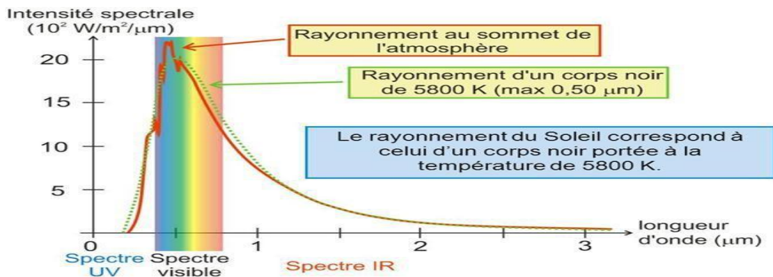
Figure I-5 : Le corps noir à 5800 °K et les spectres des rayonnements solaires [3]
