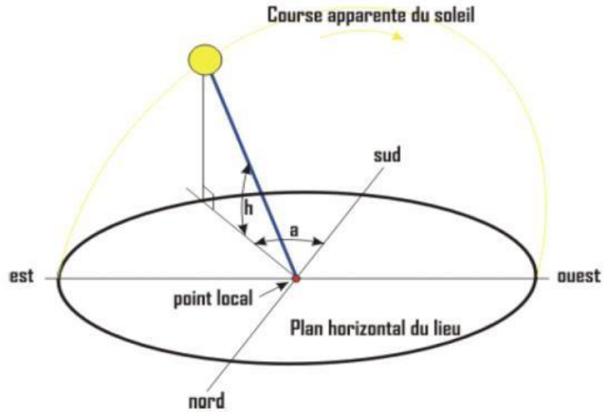
Figure I.11: Hauteur (h) ; azimut(a) du soleil [2]
