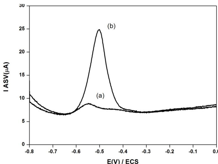
Figure IV.7 : Voltampérogrammes de SWASV a) sur CPE non modifiée (0% de Maghnite-Na) et b) sur CPE/Maghnite-Na(14%) (Après préconcentration à partir de 10^{-6} mol L -1 Pb^{2+} dans HCl 0,001M (pH=3,4) pendant t_p=5 mn sous OCP puis détection dans HCl 0,10 M (pH=1,4) ne contenant pas de Pb^{2+} ).
