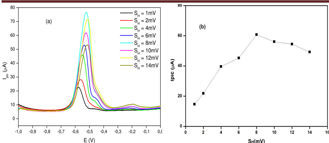
Figure IV.11 : a) Voltampérométrie de SWASV sur CPE/Maghnite-Na(14%) obtenus à partir de 10^{-6} \text{ mol L}^{-1} Pb^{2+} à différentes valeurs de hauteur d'échelon ( S_H ) et b) Variation de I_{pic} en fonction de S_H à E_d = -1,0V et aux valeurs optimales déterminées ( t_d = 15s , P_H = 50mV et P_W = 20ms ). (Mêmes conditions que la figure IV.7).
