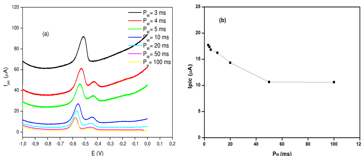
Figure IV.10 : a) Voltampérogrammes de SWASV sur CPE/Maghnite-Na(14%) obtenus à partir de 10^{-6} \text{ mol L}^{-1} Pb^{2+} à différentes valeurs de durée d'impulsion ( P_w ) et b) Variation de I_{pic} en fonction de P_w aux valeurs : E_d = -1,0V , S_H = 1mV et aux valeurs optimales déterminées t_d = 15s et P_H = 50mV . (Mêmes conditions que la figure IV.7).
