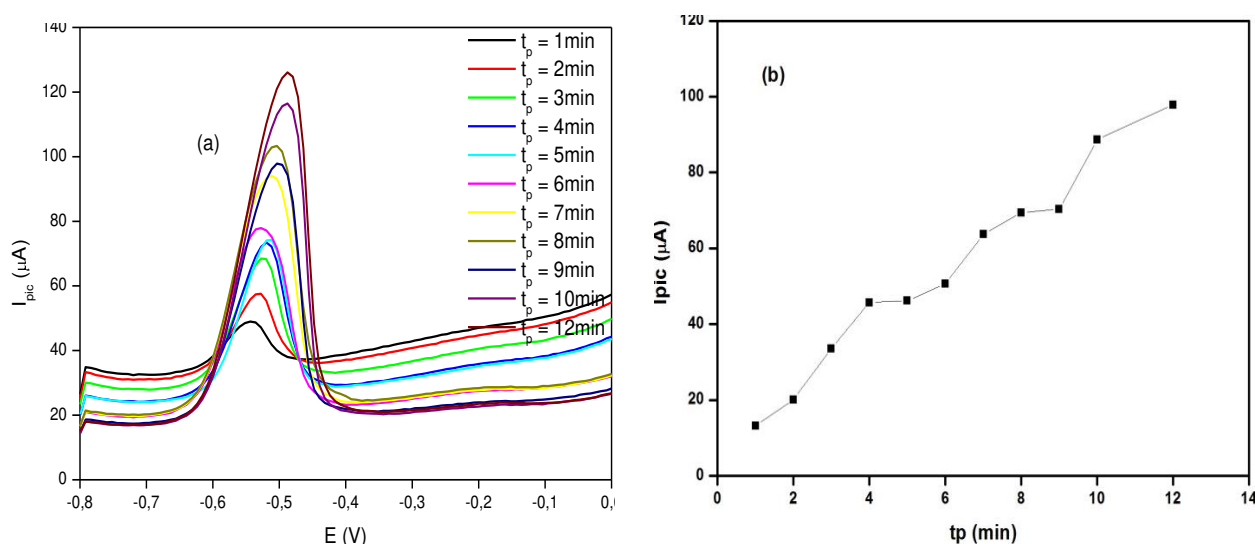
Figure IV.13 : a) Voltampérogrammes de SWASV sur CPE/Maghnite-Na(14%) obtenus à partir de 10^{-6} mol L^{-1} Pb^{2+} à différentes valeurs de temps de préconcentration ( t_p ) et b) Variation de I_{pic} en fonction de t_p aux valeurs optimales déterminées : t_d=15s , P_H=50mV , P_W=20ms , S_H=8mV et E_d=-0,8V . (Mêmes conditions que la figure IV.7).
