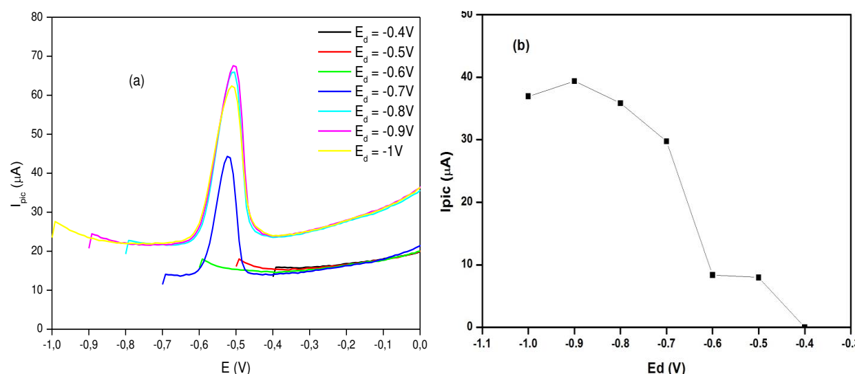
Figure IV.12 : a) Voltampérométrie de SWASV sur CPE/Maghnite-Na(14%) obtenus à partir de 10^{-6} \text{ mol L}^{-1} Pb^{2+} à différentes valeurs de potentiel de déposition ( E_d ) et b) Variation de I_{pic} en fonction de E_d aux valeurs optimales déterminées : t_d = 15s , P_H = 50mV , P_W = 20ms et S_H = 8mV . (Mêmes conditions que la figure IV.7).
