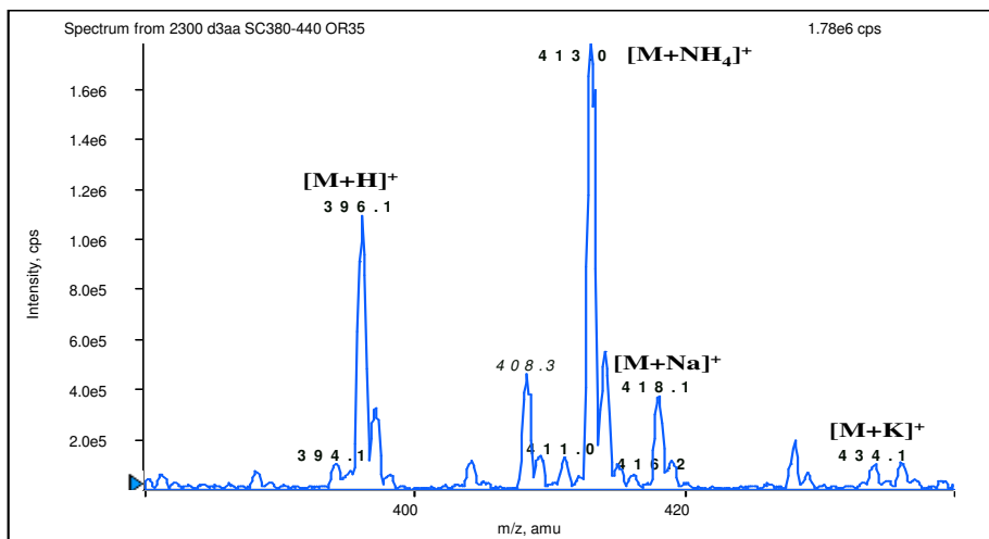
Figure 1 – Spectre de masse en mode electrospray positif de l'échantillon (46c) sur la gamme m/z 380-440. L'ion m/z 408 est issu d'une pollution présente dans le spectromètre de masse.
