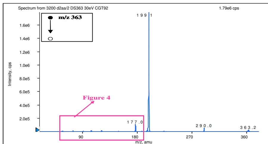
Figure 3 – Spectre des ions fragments (MS/MS) de l'ion m/z 363 ( E_{\text{collision}} : 30eV ; CGT 92).
