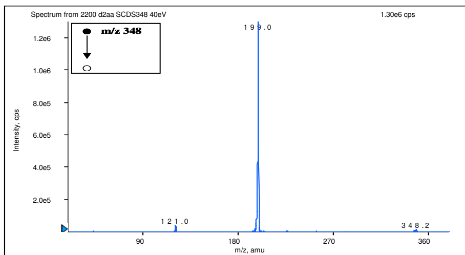
Figure 3 – Spectre des ions fragments (MS/MS) de l'ion m/z 348 ( E_{\text{collision}} : 40eV ; CGT 91).
