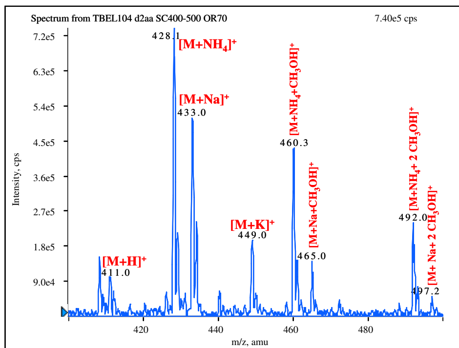
Figure 1 – Spectre de masse après ionisation electrospray en mode positif de l'échantillon ( 30a ).
