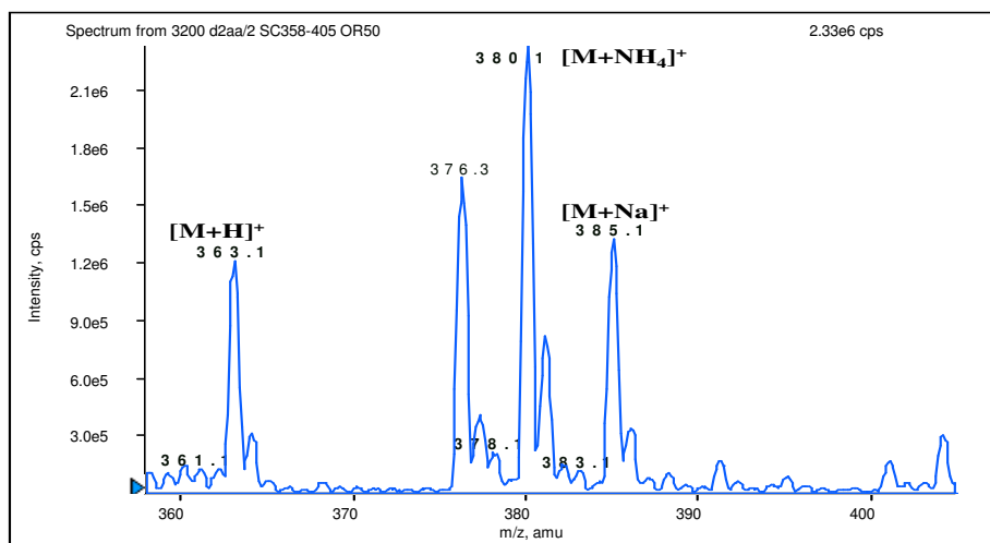
Figure 1 – Spectre de masse en mode electrospray positif de l'échantillon (30b) sur la gamme m/z 360-405. L'ion m/z 376 est issu d'une pollution présente dans le spectromètre de masse.
