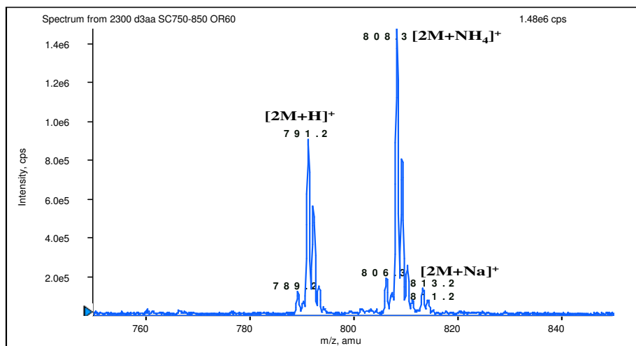
Figure 2 – Spectre de masse en mode electrospray positif de l'échantillon (46c) sur la gamme m/z 750-850.
