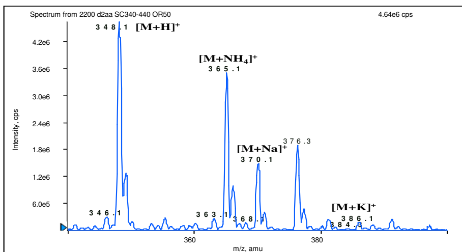
Figure 1 – Spectre de masse en mode electrospray positif de l'échantillon (46b) sur la gamme m/z 340-440. L'ion m/z 376 est issu d'une pollution présente dans le spectromètre de masse.
