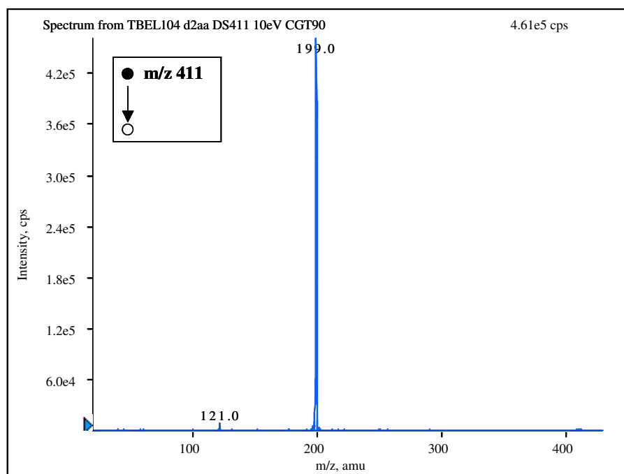
Figure 3 – Spectre des ions fragments (MS/MS) de l'ion m/z 411 ( E_{\text{collision}} : 10eV ; CGT 90).
