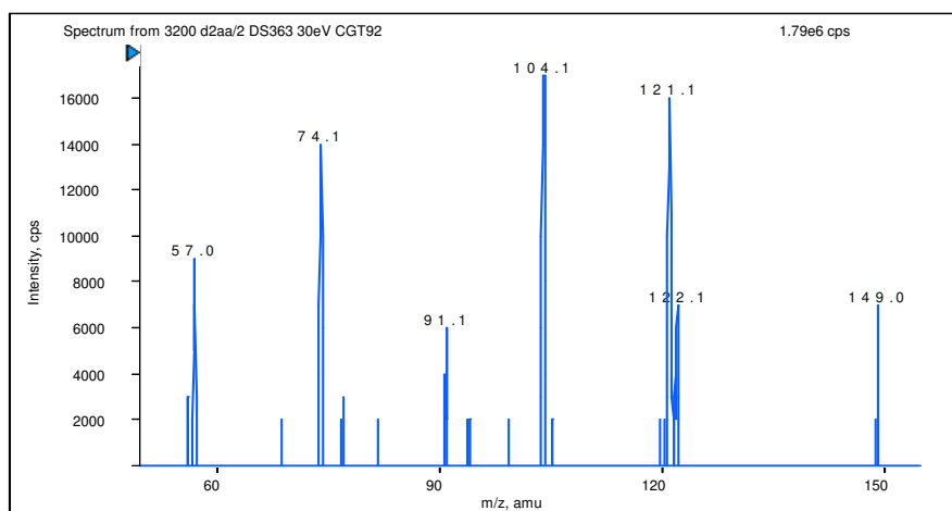
Figure 4 – Agrandissement du spectre MS/MS de l'ion m/z 363 sur la gamme m/z 55-165.
