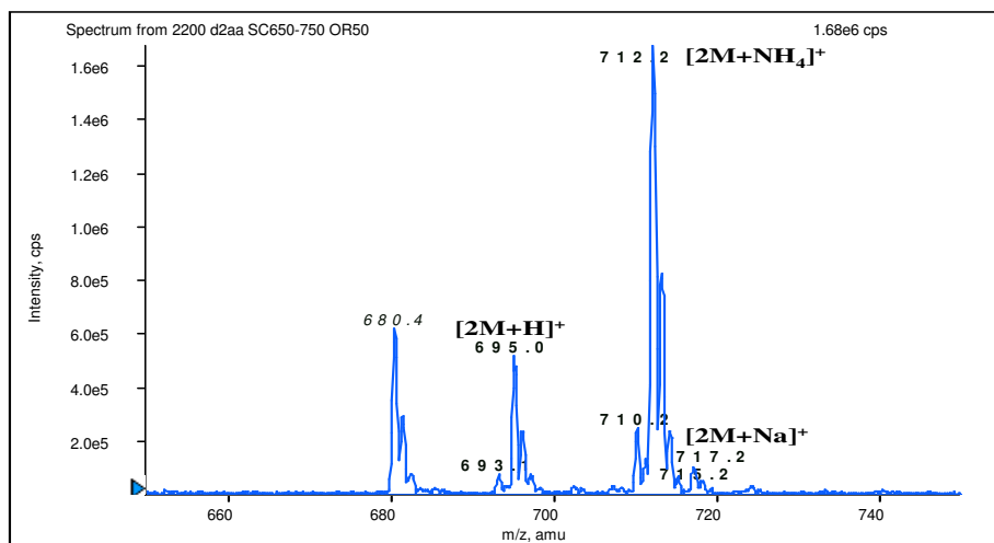
Figure 2 – Spectre de masse en mode electrospray positif de l'échantillon (46b) sur la gamme m/z 650-750. L'ion m/z 681 est issu d'une pollution présente dans le spectromètre de masse.
