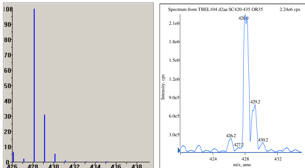
Figure 2 – Profil isotopique théorique (à gauche) et expérimental (à droite) de l'adduit ammonium du composé ( 30a ).
