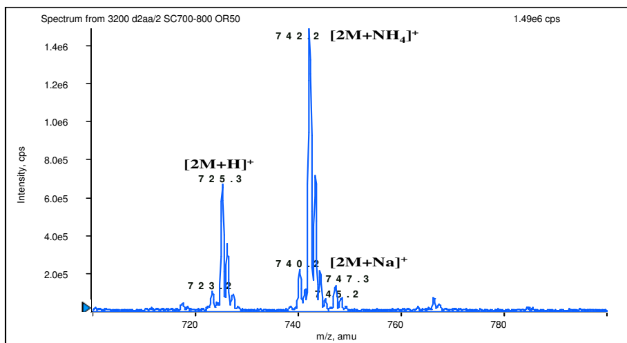
Figure 2 – Spectre de masse en mode electrospray positif de l'échantillon (30b) sur la gamme m/z 700/800.
