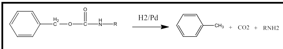
Figure 5 : Mécanisme de l'hydrogénolysation sur le palladium.
