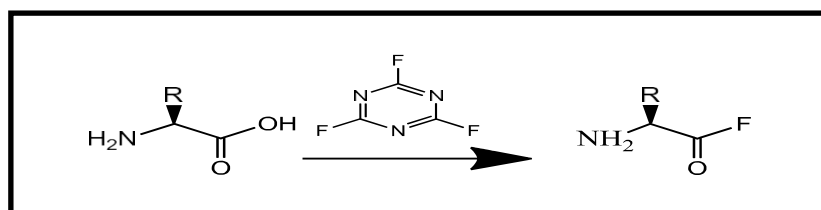
Figure 13 : Préparation d'un fluorure d'acyle.
