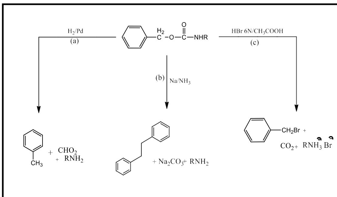
Figure 6 : les conditions de clivage du groupe benzyloxycarbonyle.
