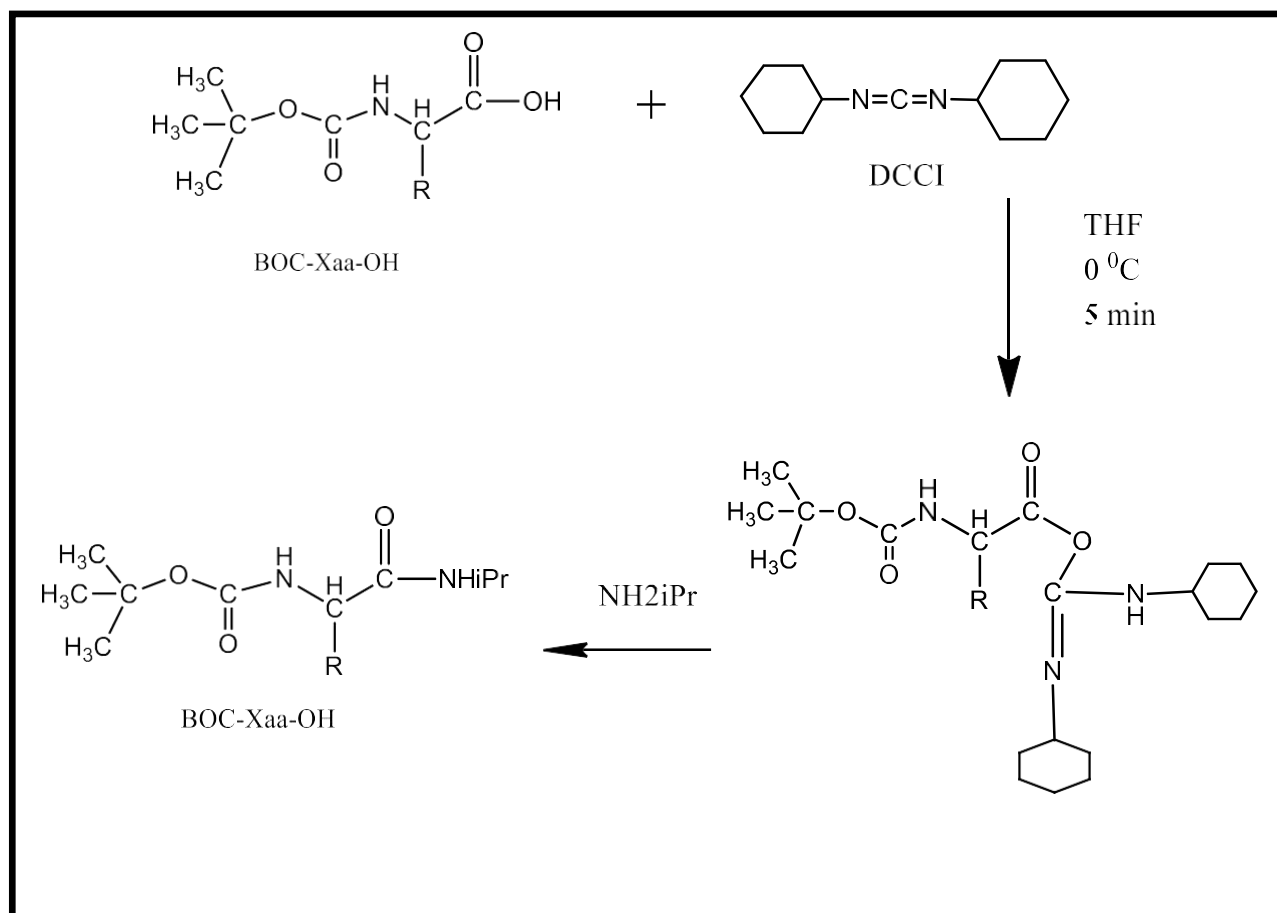
Figure 41 : Schéma général pour la synthèse des acides aminés
