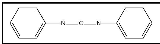
Figure 33 : Structure de DCCI.
