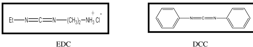
Figure 17 : Structure de DCC et EDC
