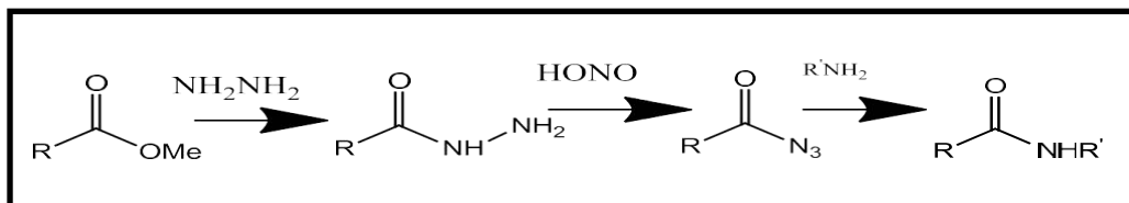
Figure 15 : Préparation des Acylazides.
