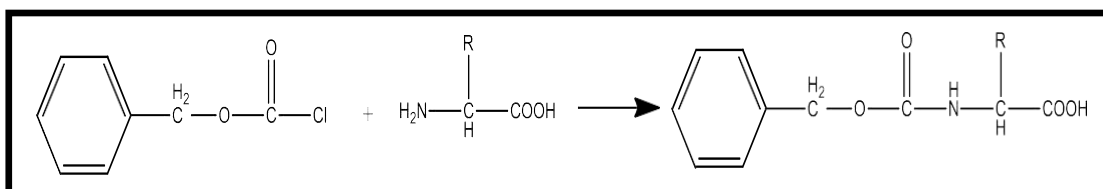
Figure 4 : Mécanisme de la protection par benzyloxycarbonyle.
