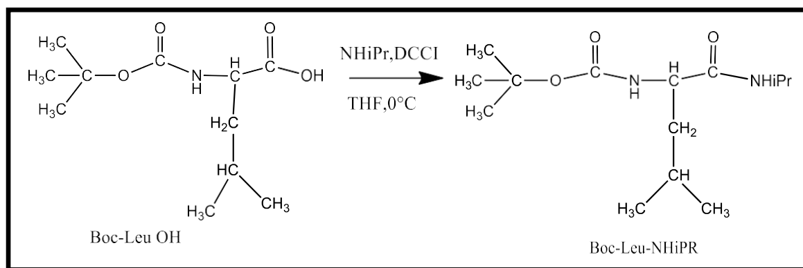
Figure 50 : Réaction de synthèse du Boc-Leu-NHiPr.
