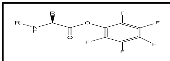
Figure19 : Pentafluorophényle (Pfp)
