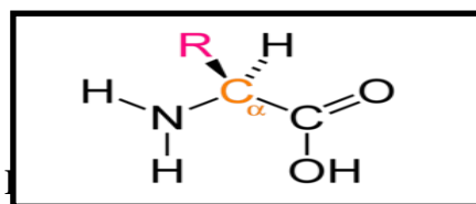
Figure 1 : Structure d'un acide aminé.
