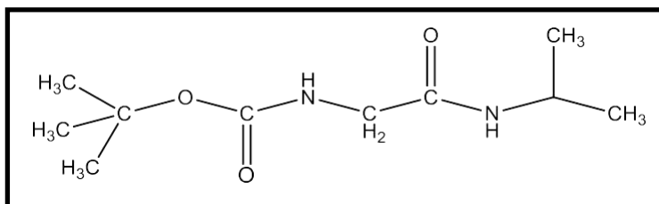
Figure 36 : Formule développée du BOC-Gly-NHiPr.
