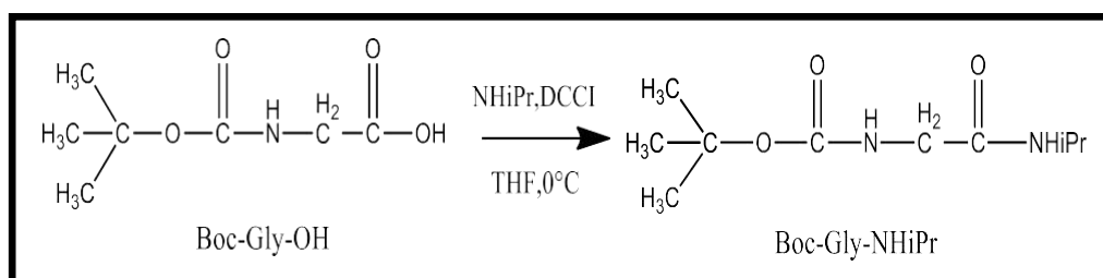
Figure 46 : Réaction de synthèse du Boc-Gly-NHiPr.
