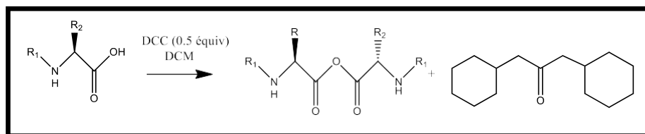
Figure 18 : Formation d'anhydride symétrique
