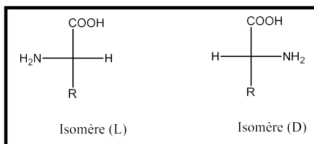
Figure 3 : Projection de Fischer des configurations D et L.
