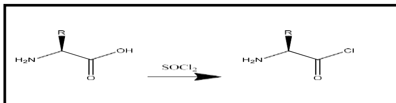
Figure 12 : Préparation d'un chlorure d'acyle.
