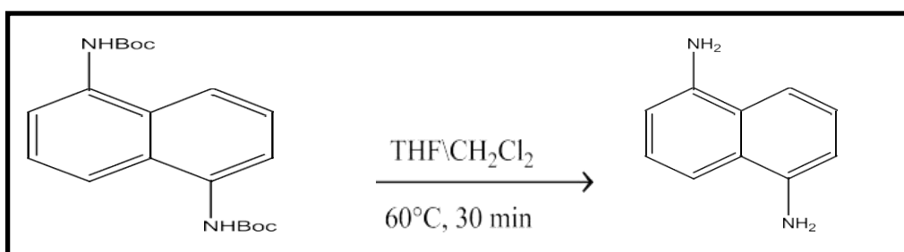
Figure 9 : Déprotection de Boc en milieu acide.
