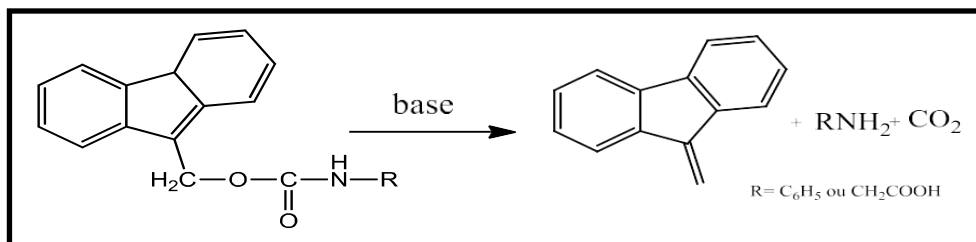
Figure 11 : Mécanisme clivage du Fmoc en milieu basique.
