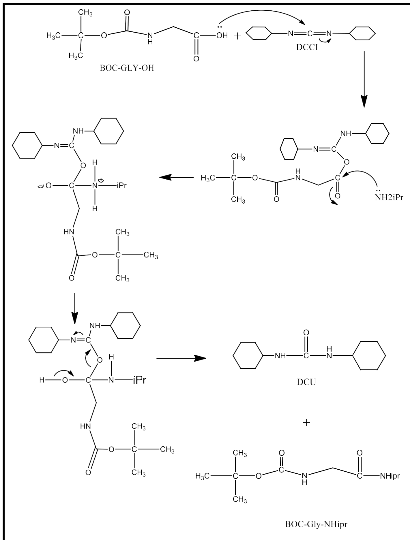
Figure 47 : Mécanisme proposé pour la synthèse du BOC-Gly-NHPr.
