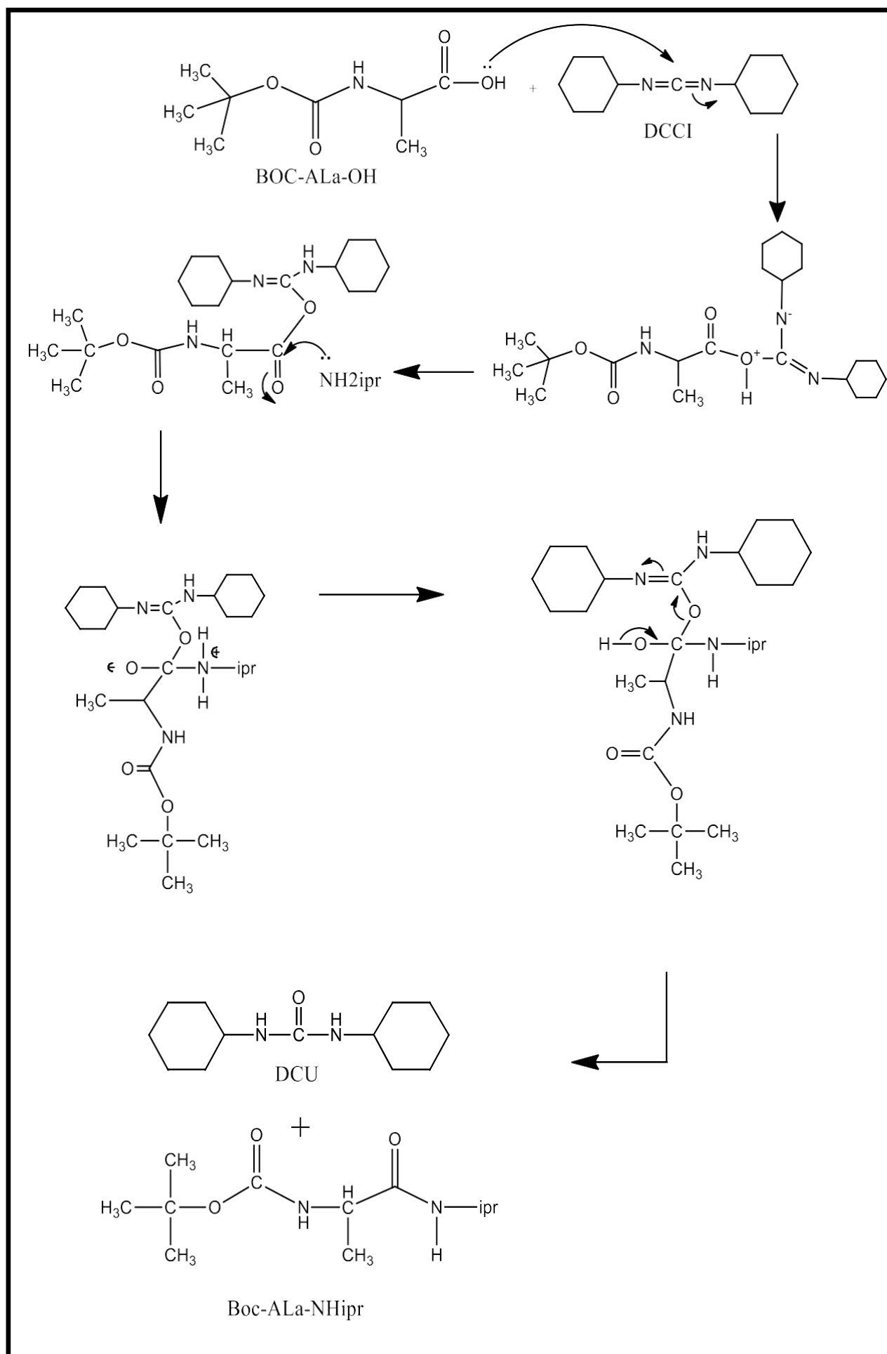
Figure 43 : Mécanisme proposé pour la synthèse du Boc-Ala-NHipr
