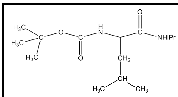
Figure 37 : Formule développée du BOC-Leu-NHiPr.
