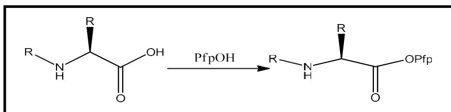
Figure 20 : Synthèse d'ester activé en présence de PfpO
