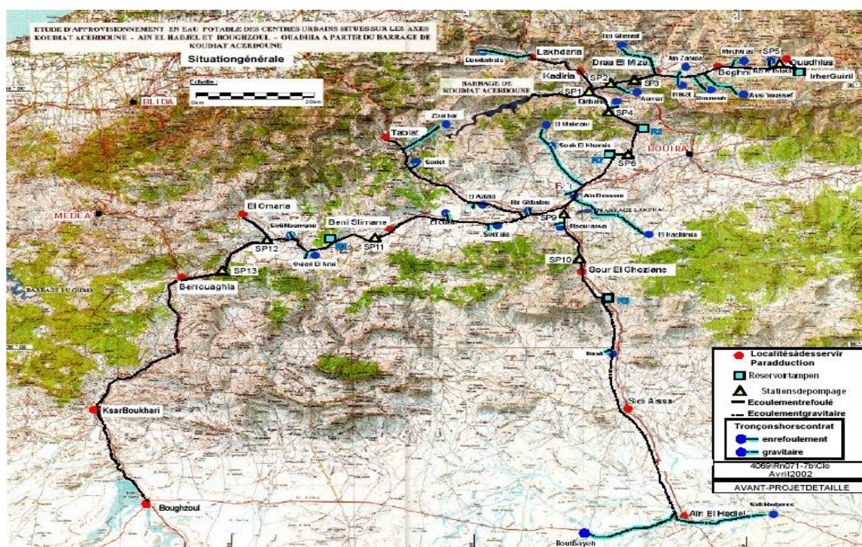
Figure IV.14 : Système de Koudiat Acerdoune-Hauts plateaux.
