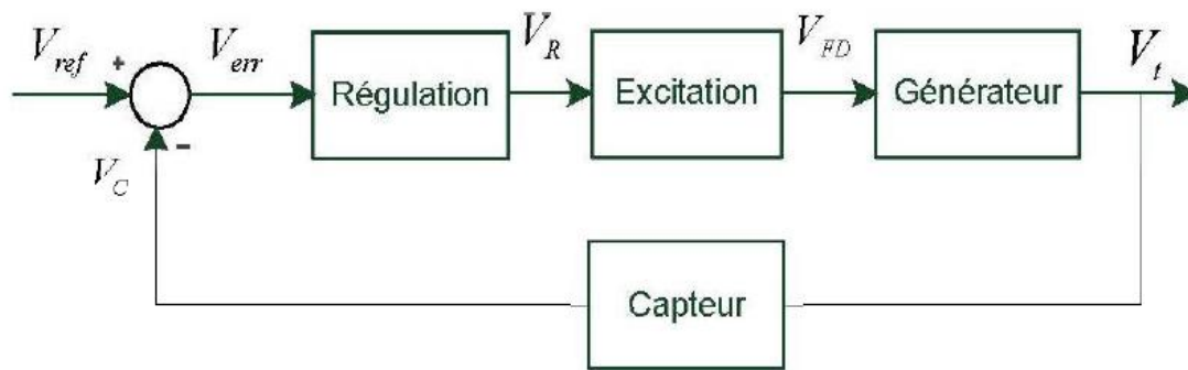
Figure I.15 : Principe de la régulation de tension dans un groupe turbine alternateur [14] [34] [35]
