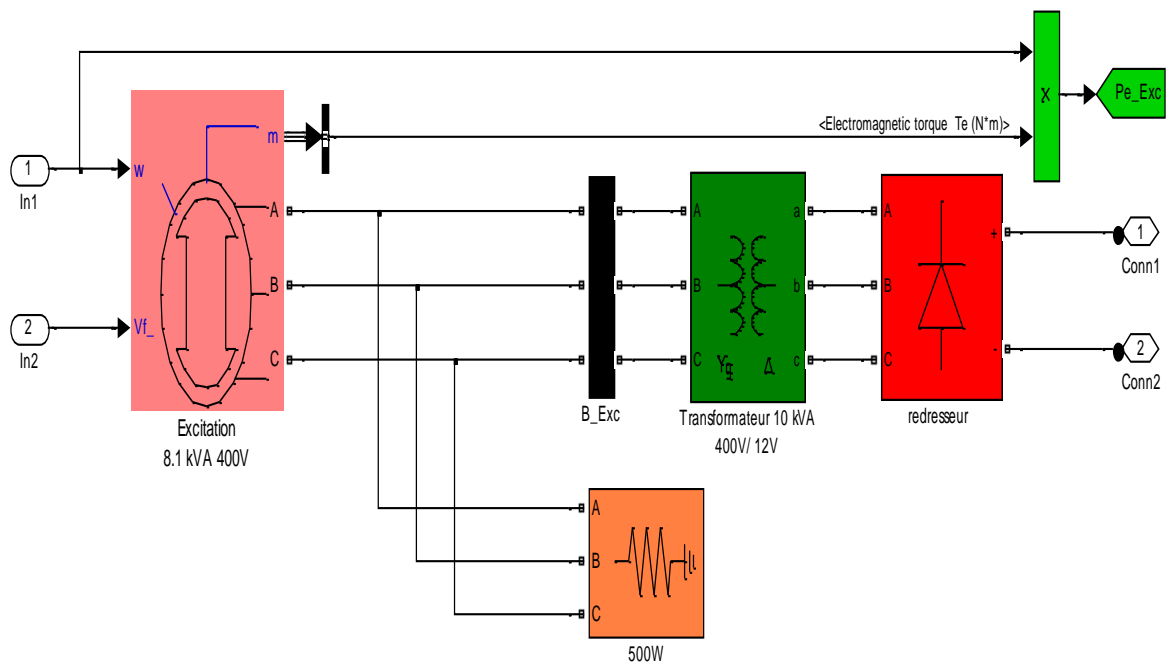
Figure III.5 :Bloc du système d'excitation
