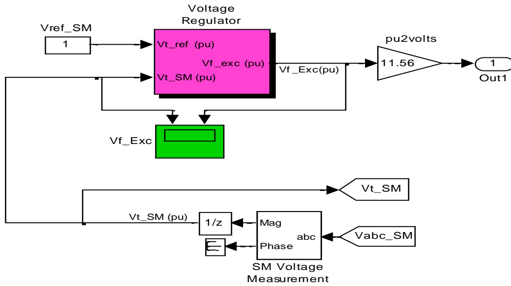
Figure III.6 :Bloc du régulateur de tension
