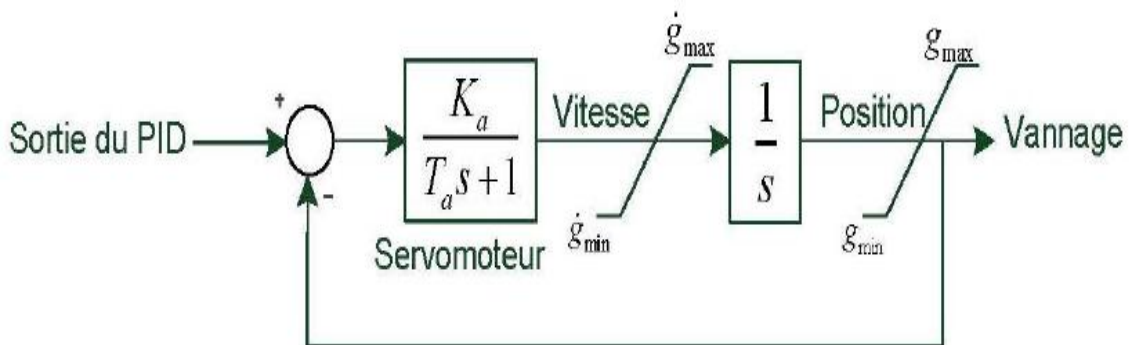
Figure I.23 : Schéma bloc du Servomoteur
