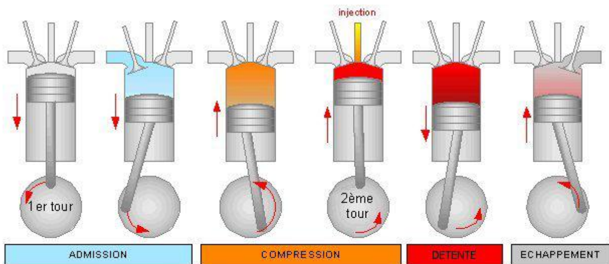
Figure II.6 : Cycle de fonctionnement d'un moteur diesel à 4 temps [39].
