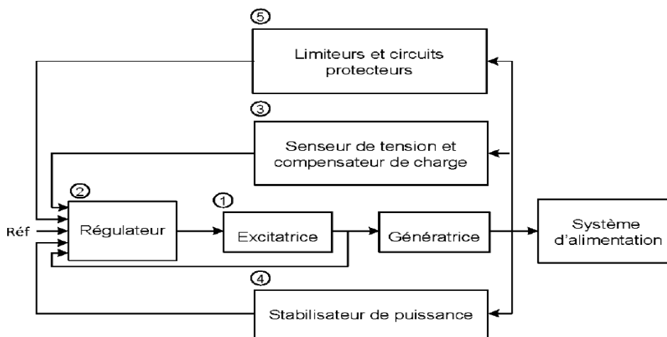
Figure I.7 : Schéma fonctionnel du système d'excitation d'une génératrice synchrone [ 14]
