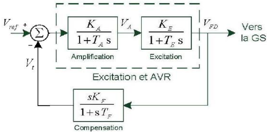
Figure I.16 : Système d' excitation type ST1 de IEEE
