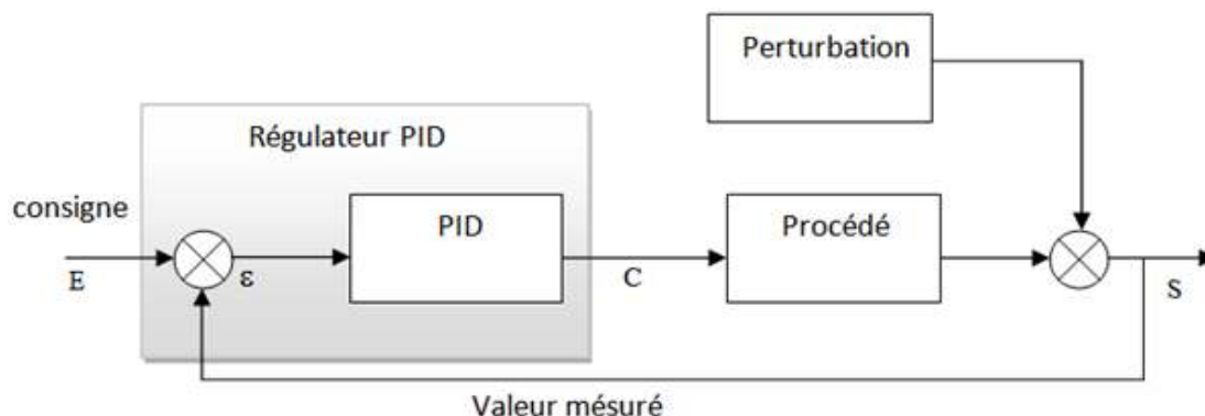
Figure I.14: Asservissement par un régulateur PID
