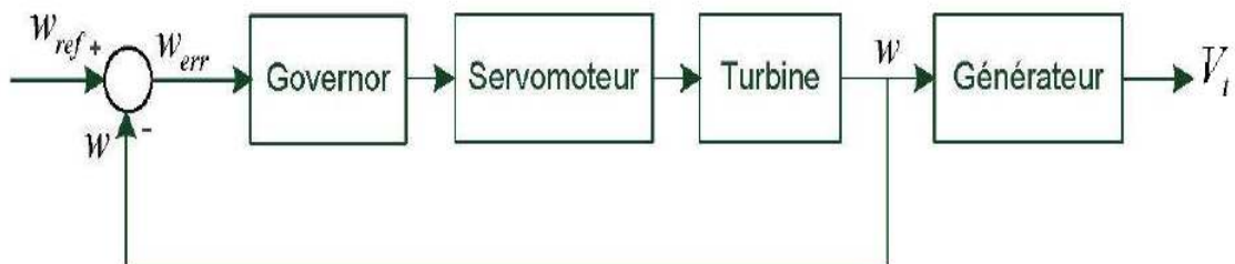
Figure I.21 : Principe de la régulation de la vitesse
