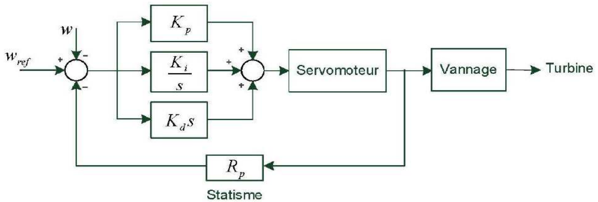
Figure I.22 : Régulateur de vitesse type PID
