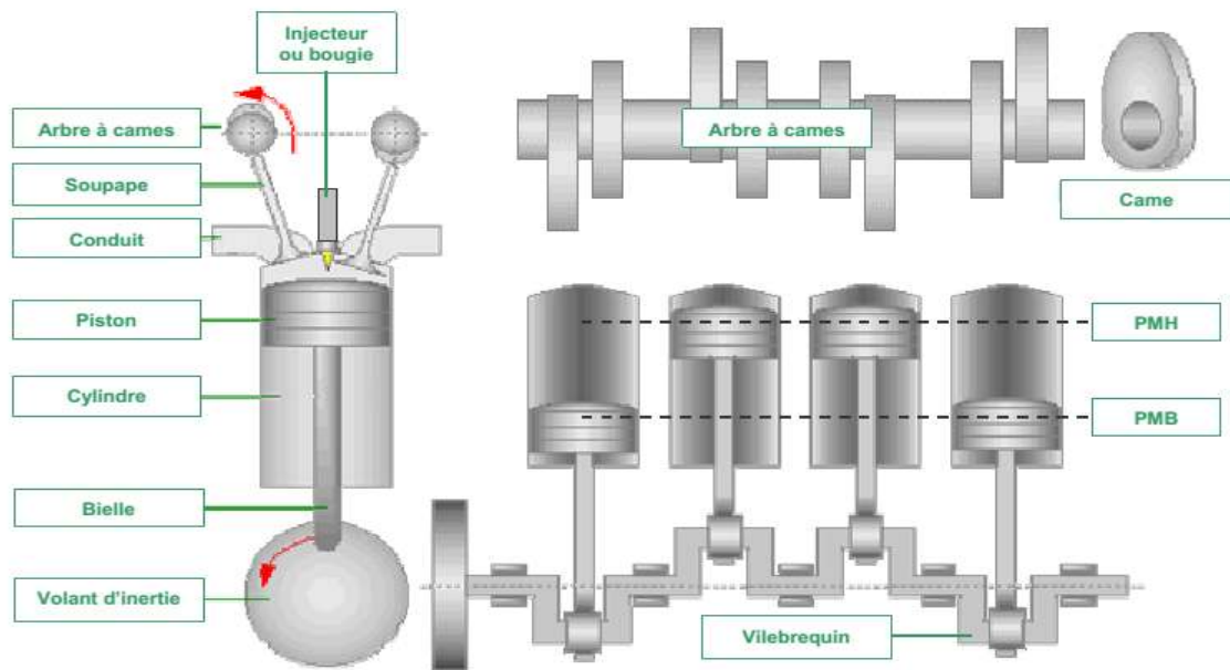
Figure II.5 : Composants principaux d'un moteur alternatif à pistons [39]
