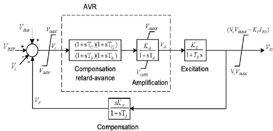
Figure I.17 : Régulation et stabilisation de la tension d'excitation
