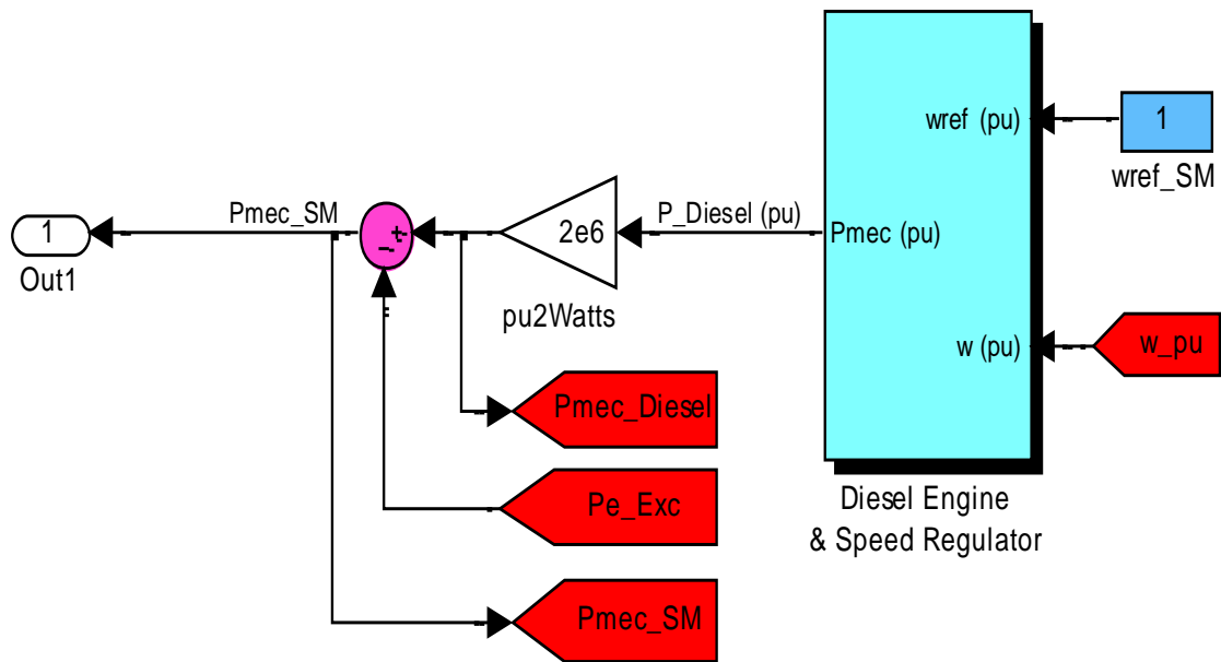
Figure III.7 :Bloc de la régulation de vitesse et le moteur diesel
