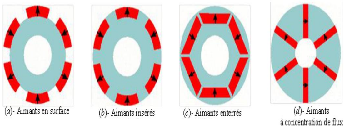
Figure I.6 : Différents structures des rotors des MSAP
