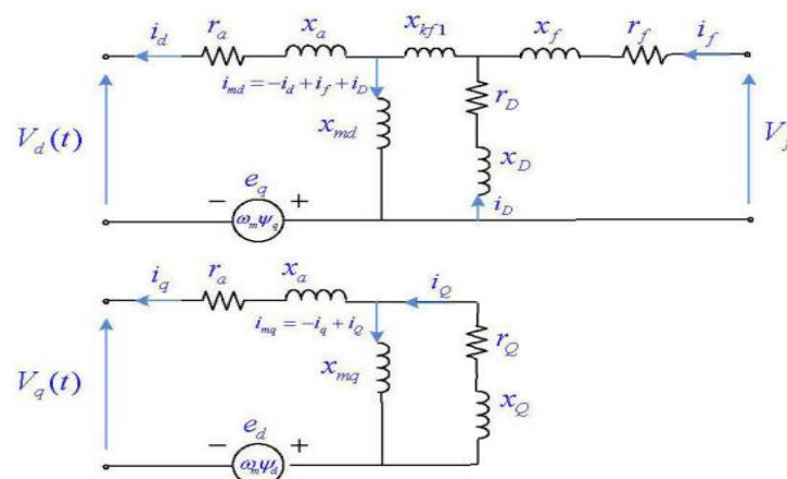
Figure II.3 : Circuits électriques équivalents de la génératrice synchrone triphasée dans le repère de Park (en pu)
