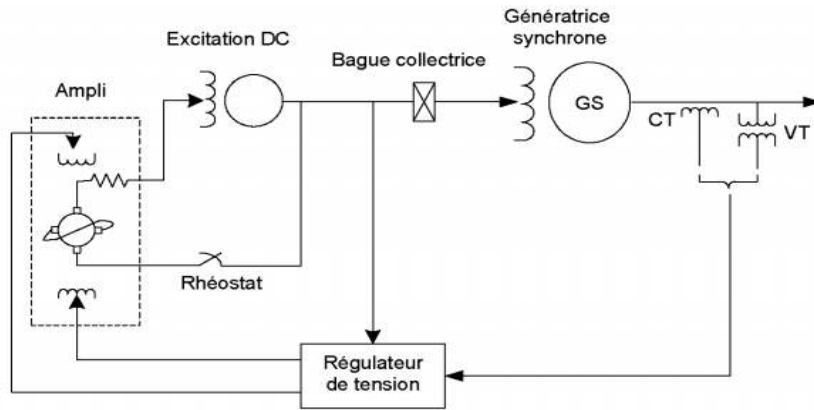
Figure I.8 : Système d'excitation de type DC
