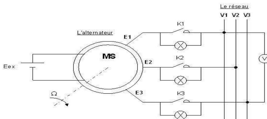
Figure I.13 : Couplage d'une machine synchrone sur un réseau [9]
