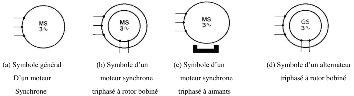
Figure I.1 : Symboles de la machine synchrone
