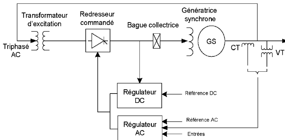
Figure I.12 : Excitatrice statique par redresseur commandé à source de tension [14]
