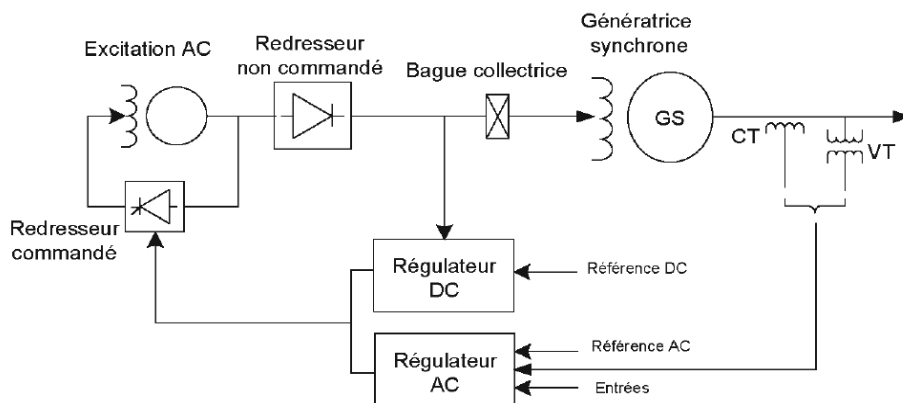
Figure I.9 : Excitation de type AC avec redresseur non commandé
