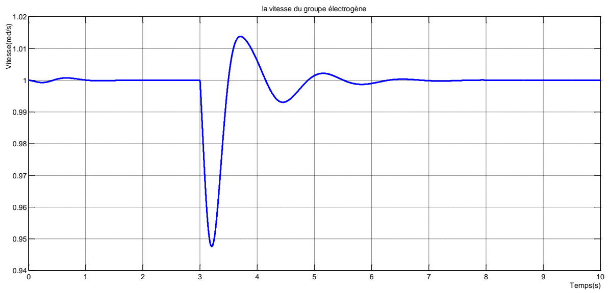
Figure III. 12 : La vitesse du groupe électrogène.
