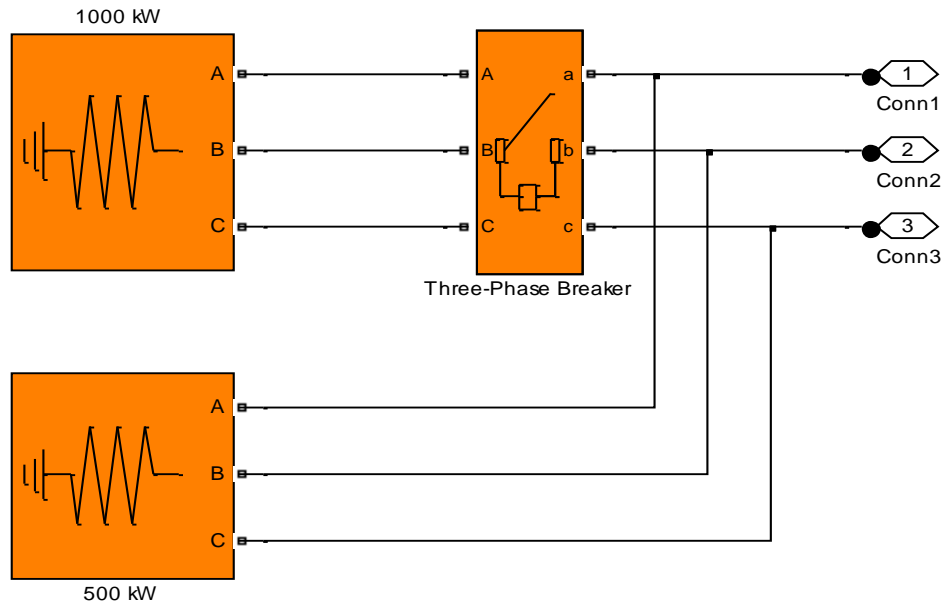
Figure III.4 :Bloc de la Charge électrique
