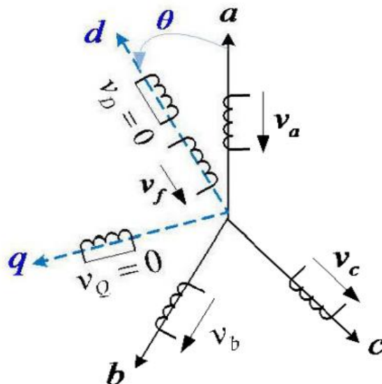
Figure II .1 : Enroulements d'une machine synchrone triphasée (repère abc)
