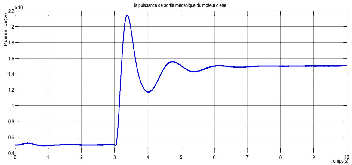
Figure III.11 : la puissance de sortie mécanique du moteur diesel.
