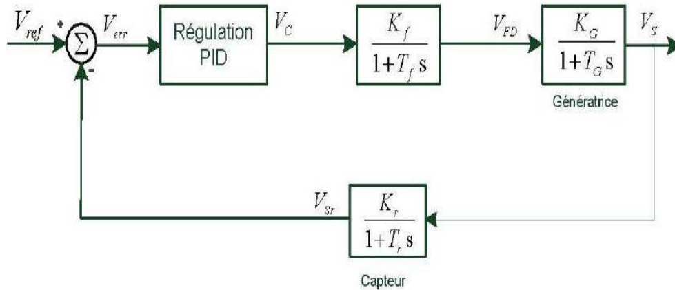
Figure I.20 : Schéma de régulation de tension simplifié
