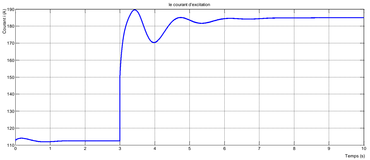
Figure III.8 :le courant d'excitation
