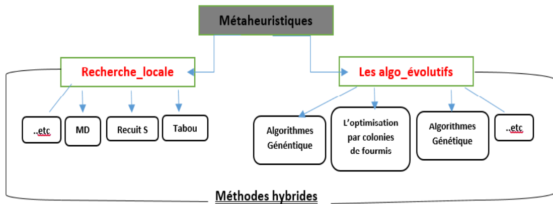
FIGURE 2.6 – Les méta-heuristiques.
