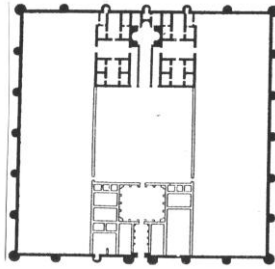
( شكل : 15 ) مخطط قصر الطوبة — عن : فريد شافعي ( شكل : 16 ) مخطط قصر المشتى — عن : كريزويل
