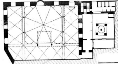
مخطط جامع صفر - عن : دوكالي .
