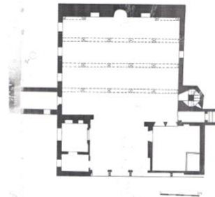
مخطط الجامع خارج القصبة - عن : دوكالي .
