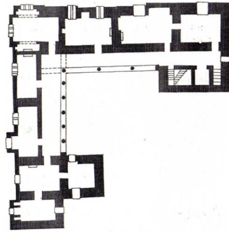
(شكل: 25). مخطط الطابق الأول .
