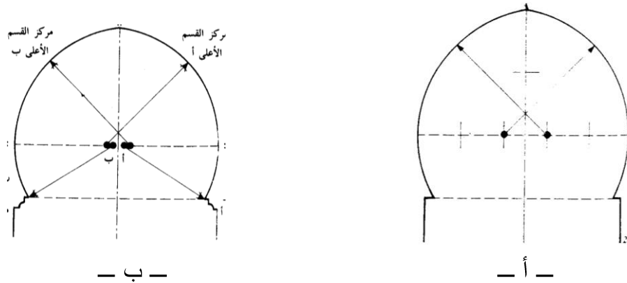
(شكل 52: تشكيل العقد المتجاوز المنكسر أ بمركزين ب بأربعة مراكز)
