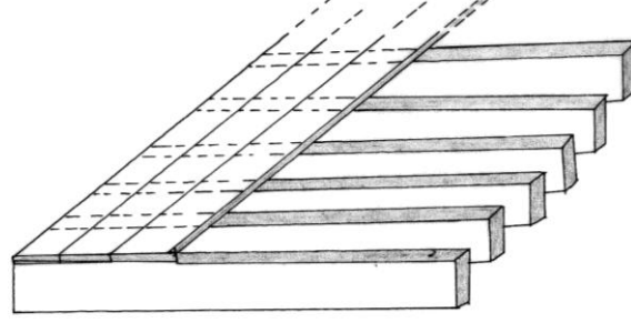
( شكل: 54 ) نموذج يوضح تركيب طبقات الأسقف المستوية
