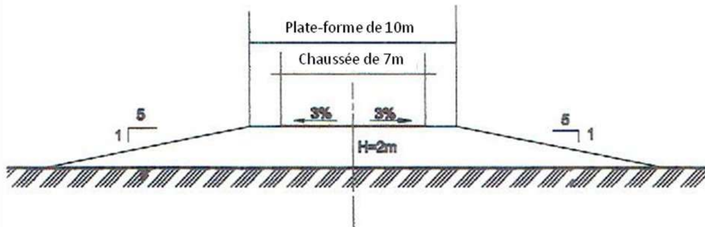
Figure 6b Profil d'équilibre de la route sans protection, la pente de la chaussée a été de 1/5 (ECH : 1/200)
