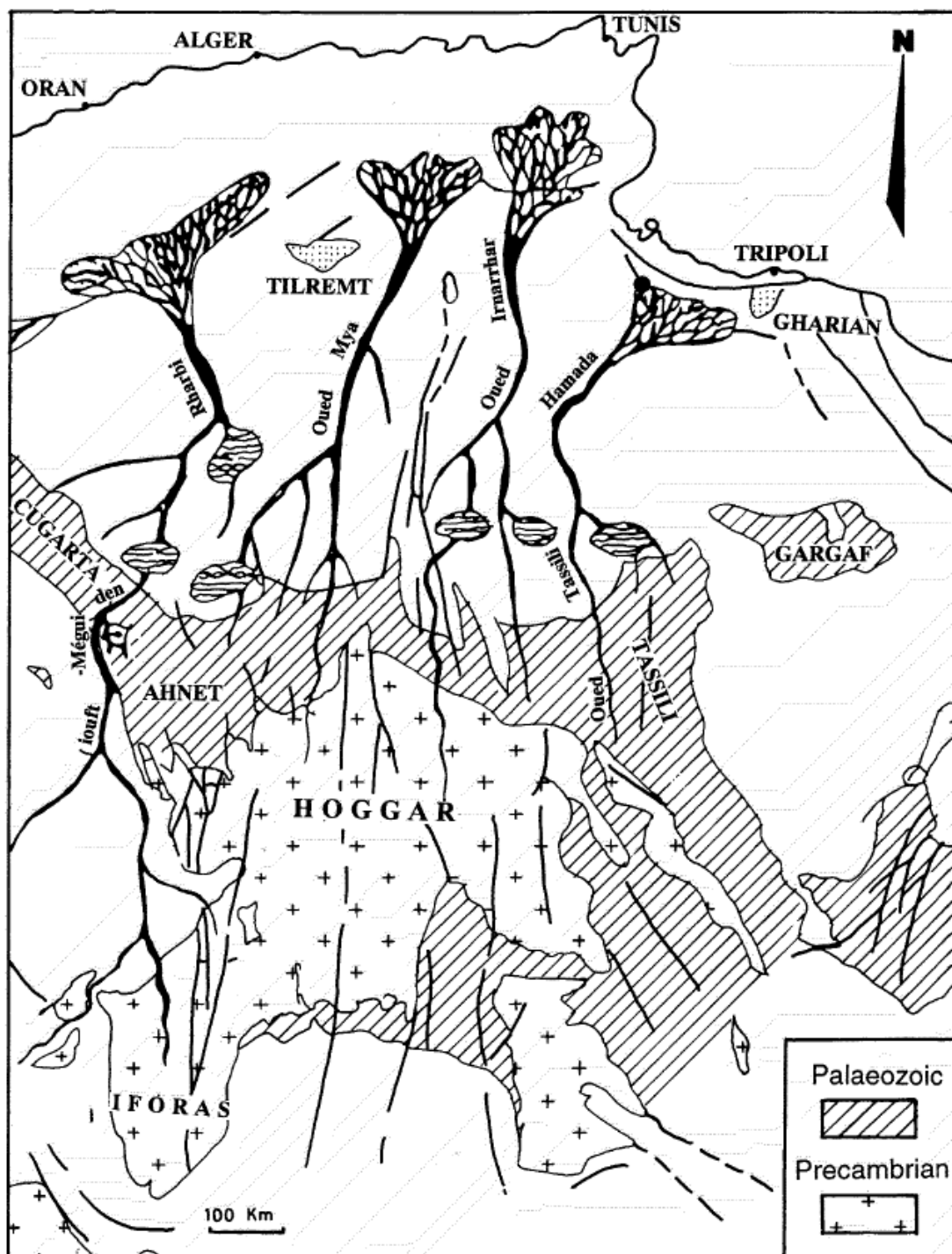
Figure 55. Origine des sables du Grand Erg Oriental (d'après Legrand et Guiraud, 1990 in Ouaja, 2003).
