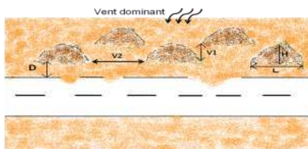
Figure 34. Drâas déposés perpendiculairement à la direction du vent dominant (d'après Sebaa et al., 2015)
