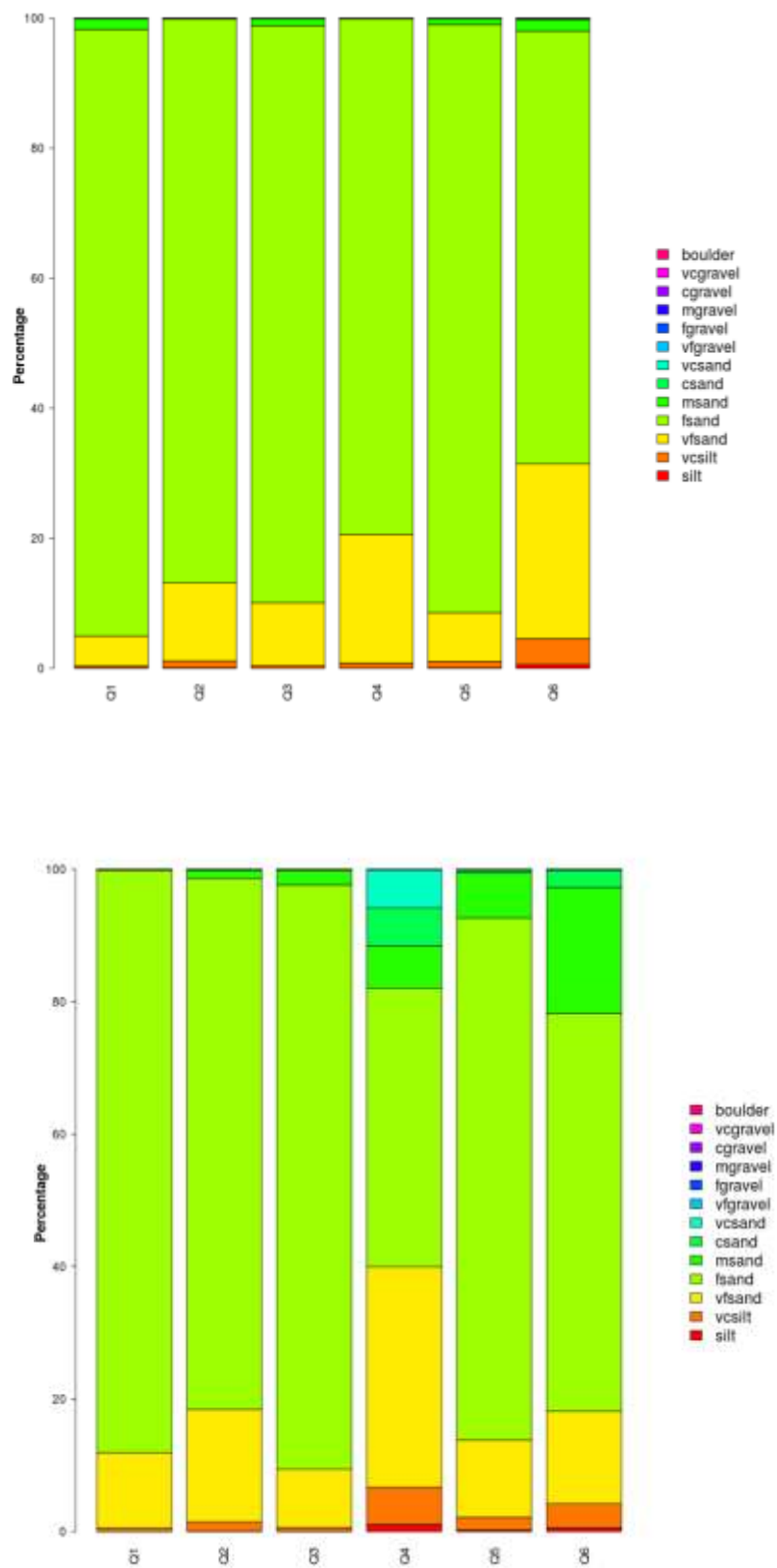
Figure 52. Les sédiments de surface au Bas-Sahara présentent un faciès sableux (d'après Sebaa, 2016).
