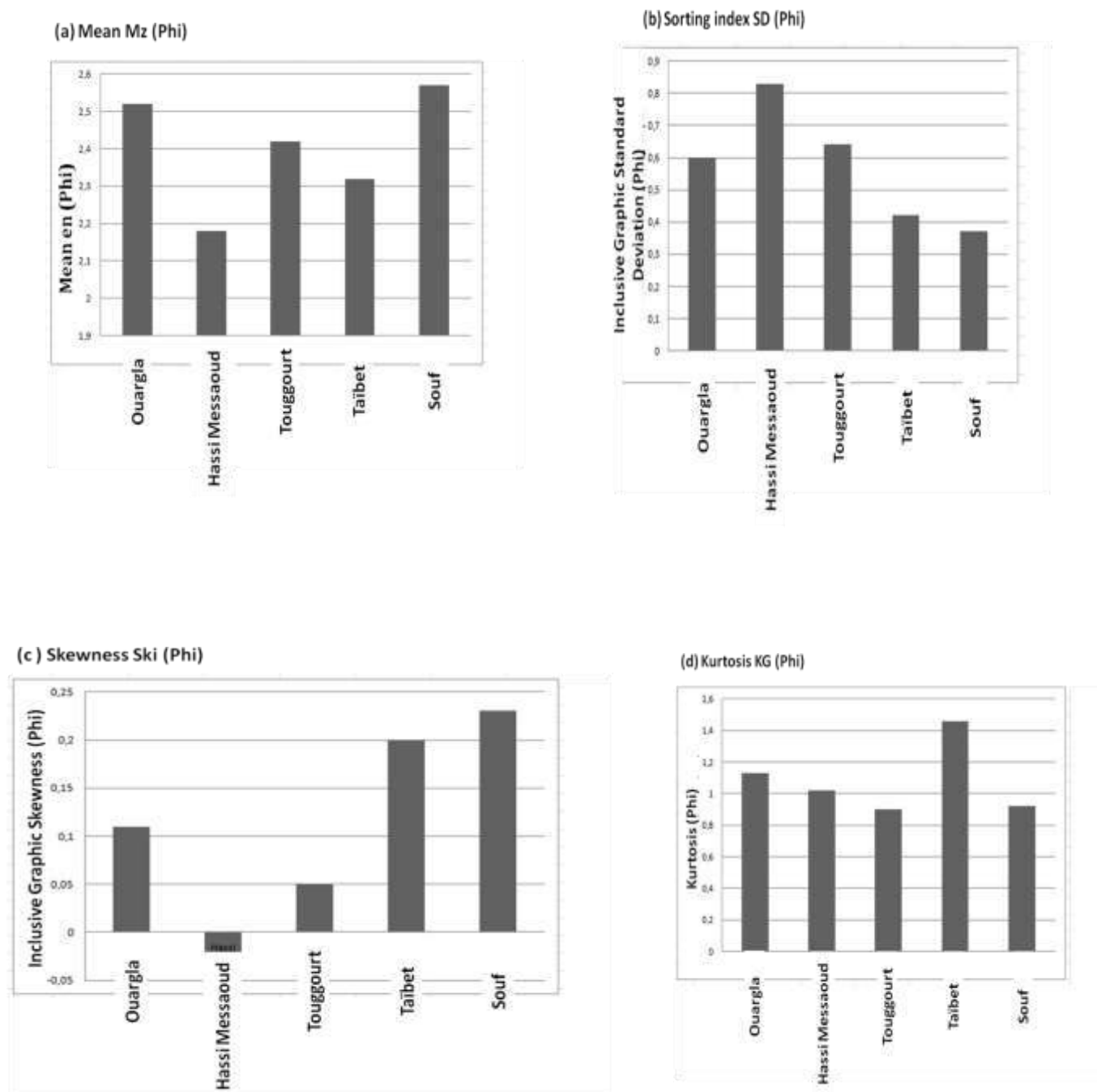
Figure 53. Valeurs moyennes des paramètres statistiques de la taille des grains, Bas-Sahara Algérien, (a) moyenne ; (b) indice de classement Sorting ; (c) coefficient d'asymétrie Skewness ; (d) coefficient d'acuité Kurtosis (d'après Sebaa, 2016)
